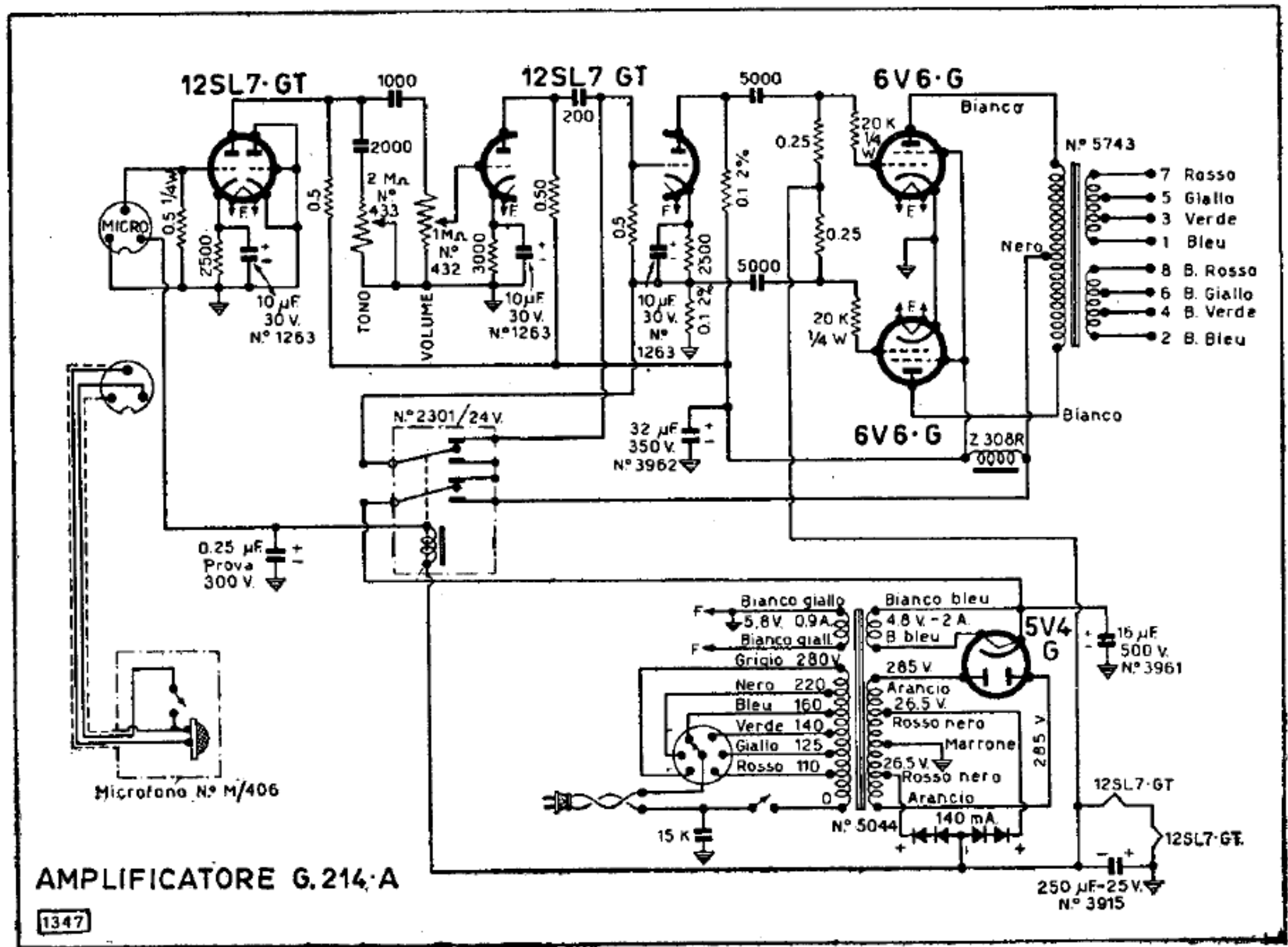
Lo schema elettrico del G.214/A.
